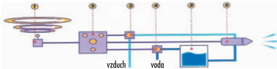
1) Vlhkoměr, 2) řídicí skříň, 3 a 4) hlavní ventily, 5) konstantní hladina vody, 6) trysky
